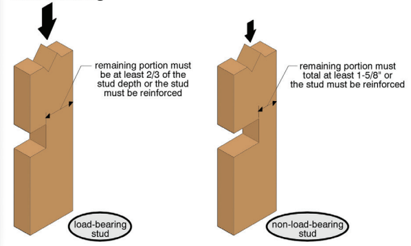
Stud notching
